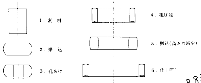
図4 リングローリングの一例
